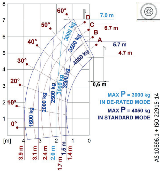
TF42.7-115EE
